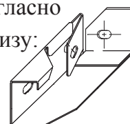
Начальное положение элемента жесткости - "лапки"
