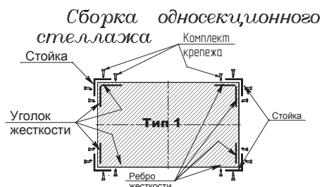
Сборка односекционного стеллажа
