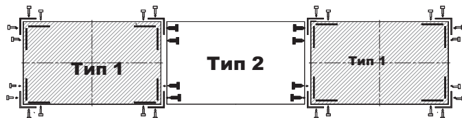
Сборка трехсекционного стеллажа
