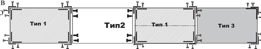
Сборка четырехсекционного стеллажа
