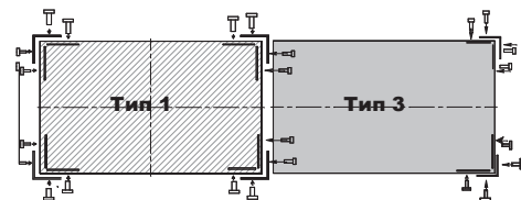
Сборка двухсекционного стеллажа
